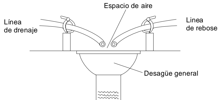
Figura 4. Línea de drenaje
